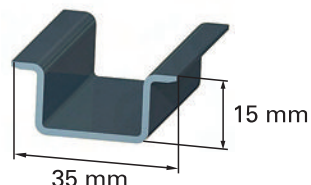
TH 35-15 x 1,5
